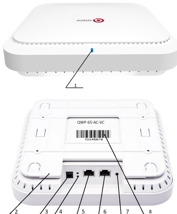
Рисунок 1. Внешний вид QWP-65-AC-VC
