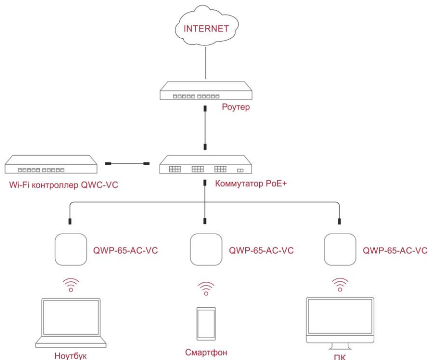
Рисунок 2. Типовая схема подключения точки доступа к сетевому оборудованию
