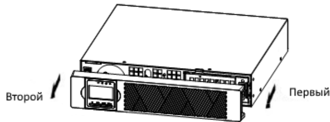
Рисунок 11. Снятие передней крышки батарейного модуля
