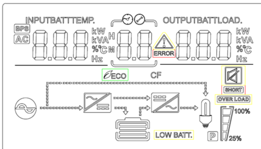
Рисунок 18. Индикаторы на ЖК-дисплее
