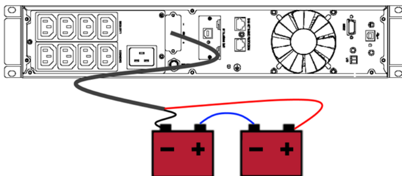
Рисунок 13. Подключение внешних аккумуляторных батарей
