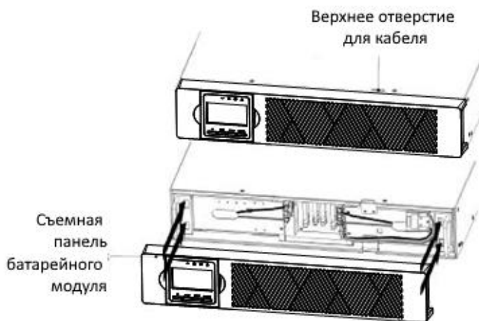
Рисунок 10. Установка передней крышки ИБП
