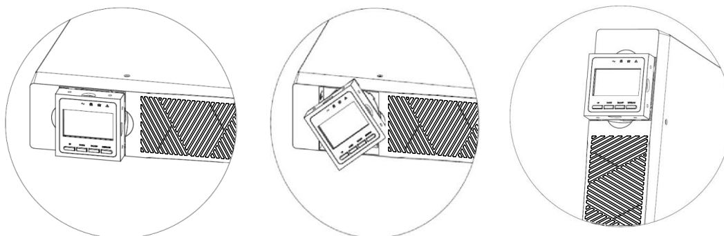
Рисунок 16. Установка дисплея для вертикального использования
