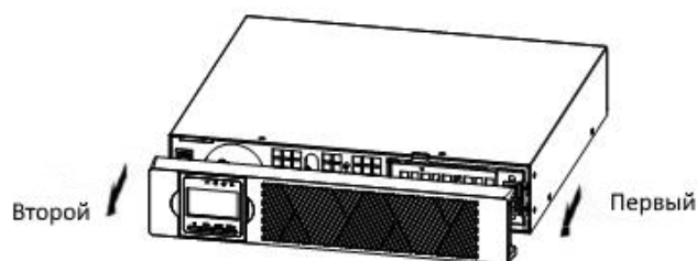
Рисунок 8. Снятие передней крышки ИБП
