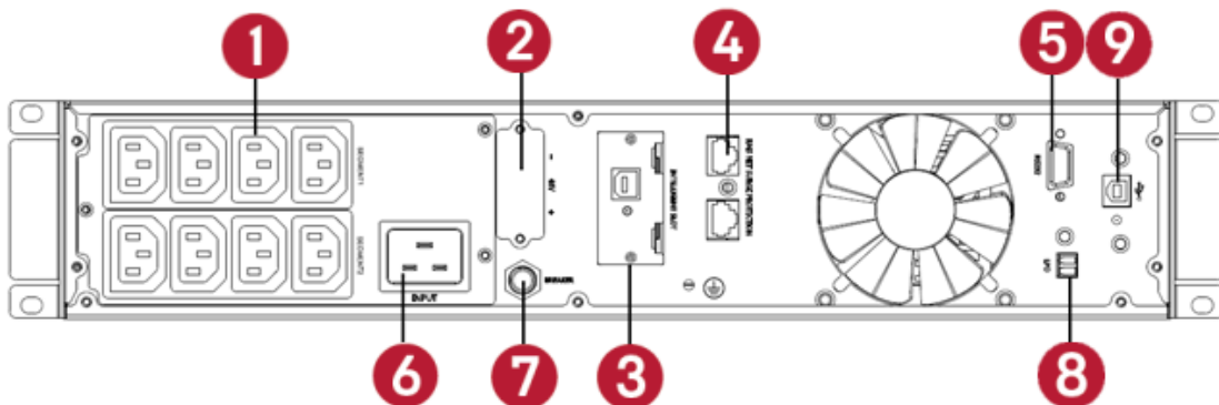
Рисунок 1. Вид задней панели ИБП 1 кВ·А и 1,5 кВ·А
