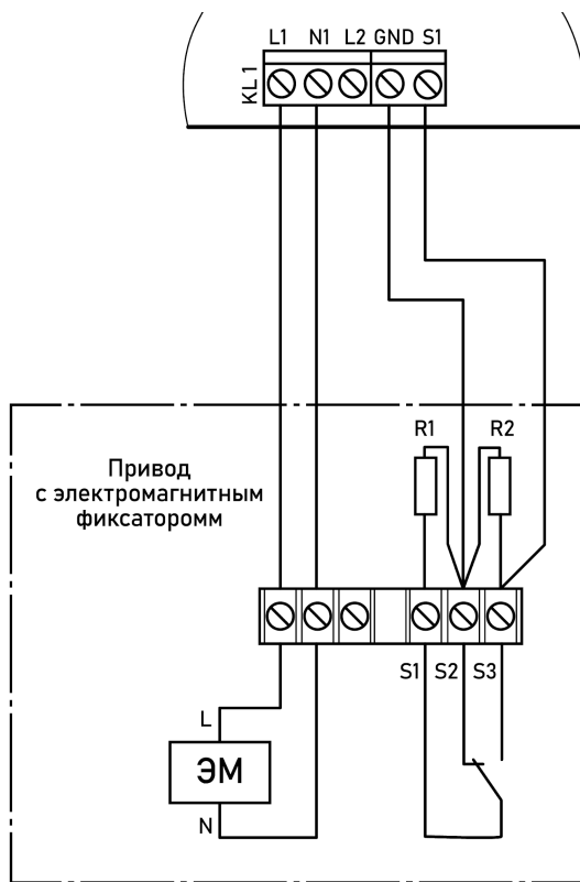
Рисунок 7 - Схема подключения привода с электромагнитным фиксатором
