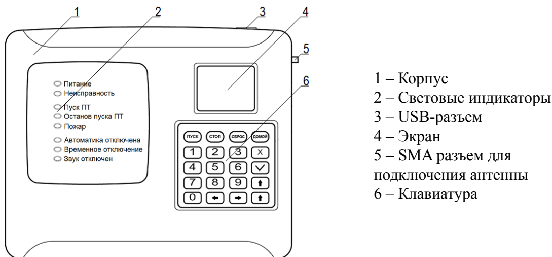
Рисунок 1 - Внешний вид ППК
