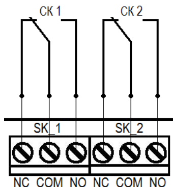
Рисунок 11 - Схема подключения к СК прибора
