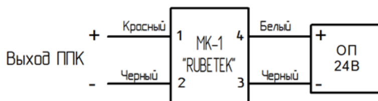
Рисунок 10 - Схема подключения МК-1 к ОП
