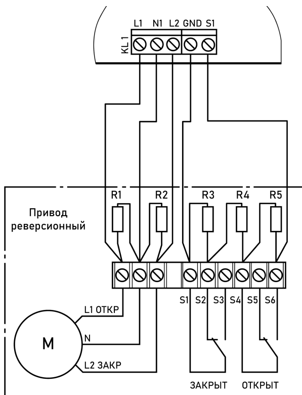
Рисунок 6 - Схема подключения реверсивного привода
