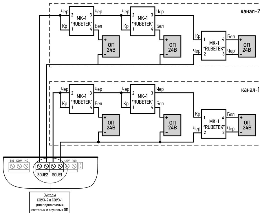
Рисунок 9 - Схема подключения СОУЭ
