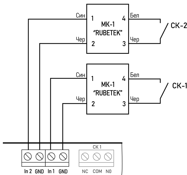
Рисунок 12 - Схема подключения свободно программируемых входов
