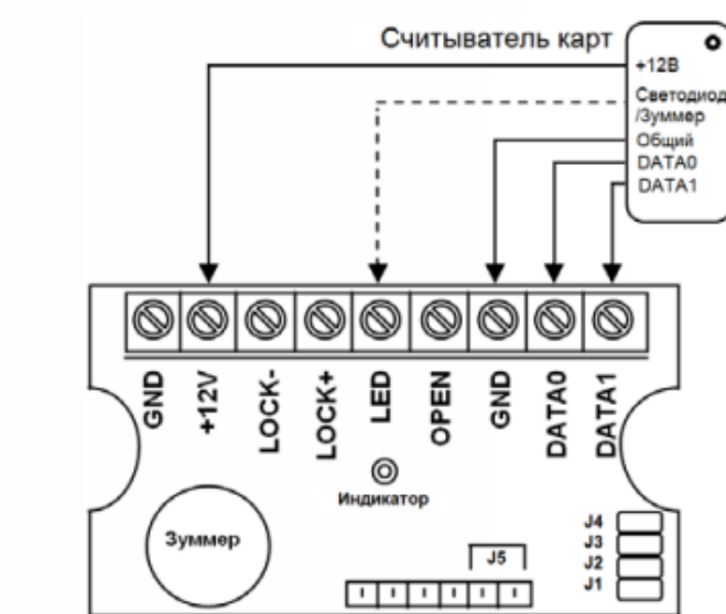
Рисунок 3. Общая схема подключения на примере OPTIMUS SK-01
