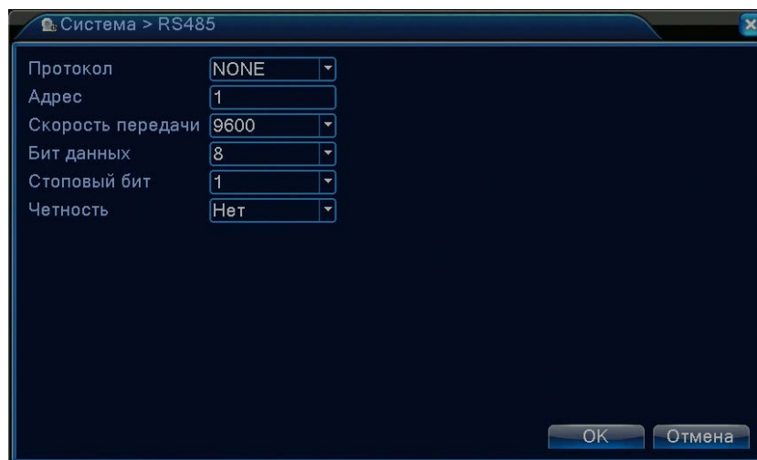
Рисунок 4.33 Конфигурация RS485 устройств в цифровом режиме.
