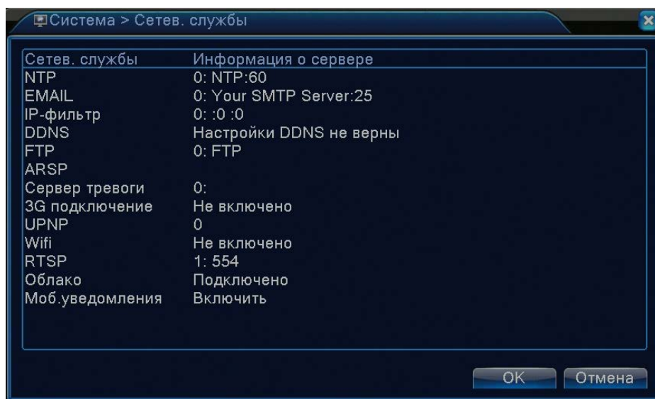
Рисунок 4.17 Сетевые службы
