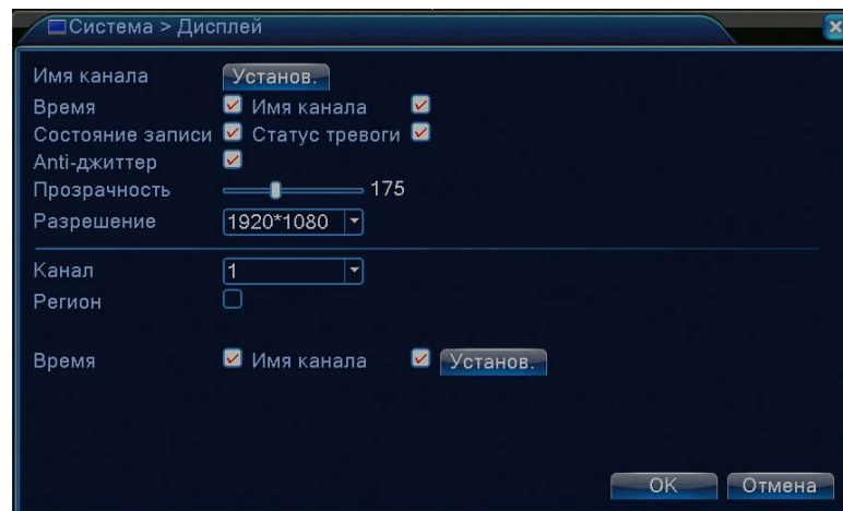
Рисунок 4.30 Настройки дисплея
