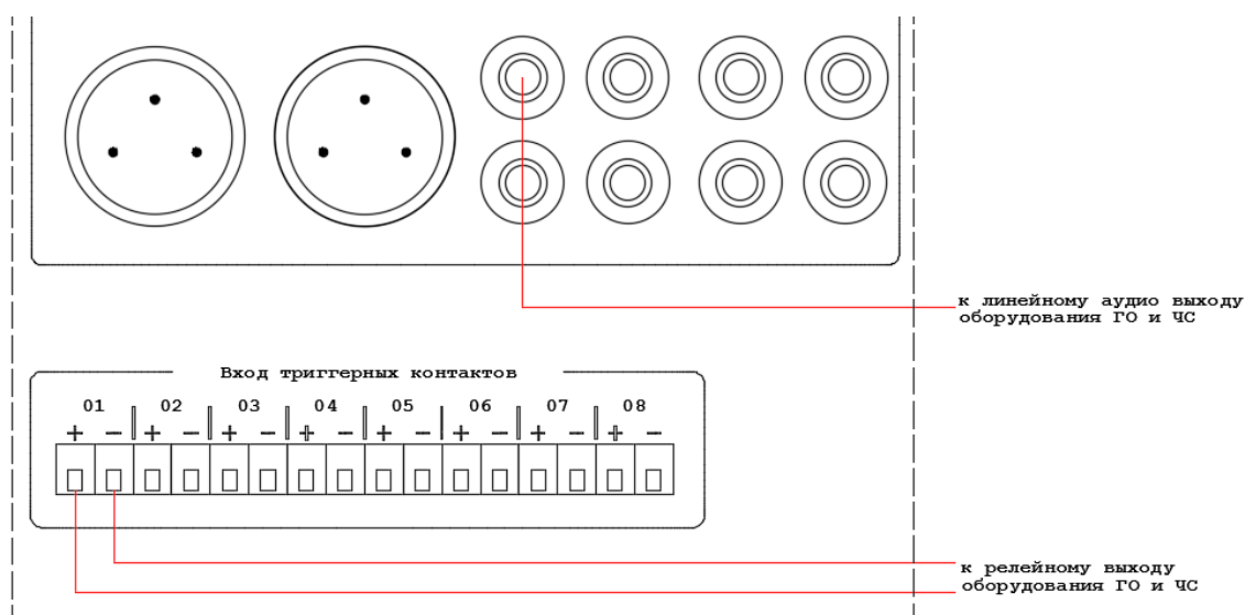
Рис. 3.9. Схема подключения сигналов ГО и ЧС к LPA-PRESTA-16.
