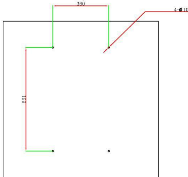
Рис. 3.7.1. Монтажные отверстия для LPA-Presta-16
