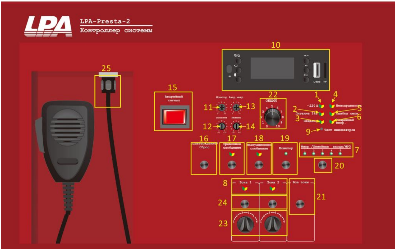
Рис. 2.1. Контроллер системы LPA-PRESTA-2 (передняя панель)
