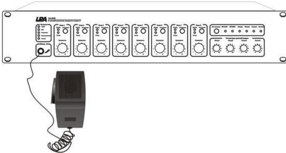
Рис. 4.2. Схема подключения микрофона для экстренных сообщений к разъему «Микр. 1» на лицевой панели усилителя мощности LPA-EVA-8500
