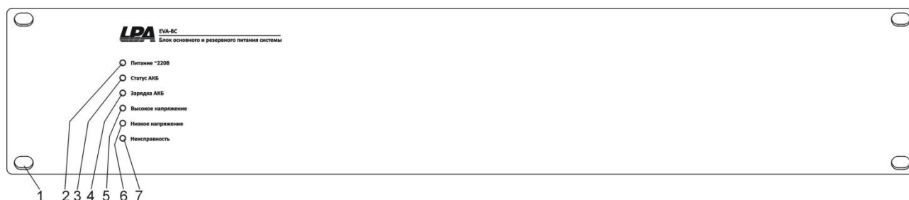
Рис. 3.2. Лицевая панель резервного источника питания и зарядного устройства LPA-EVA-BC
