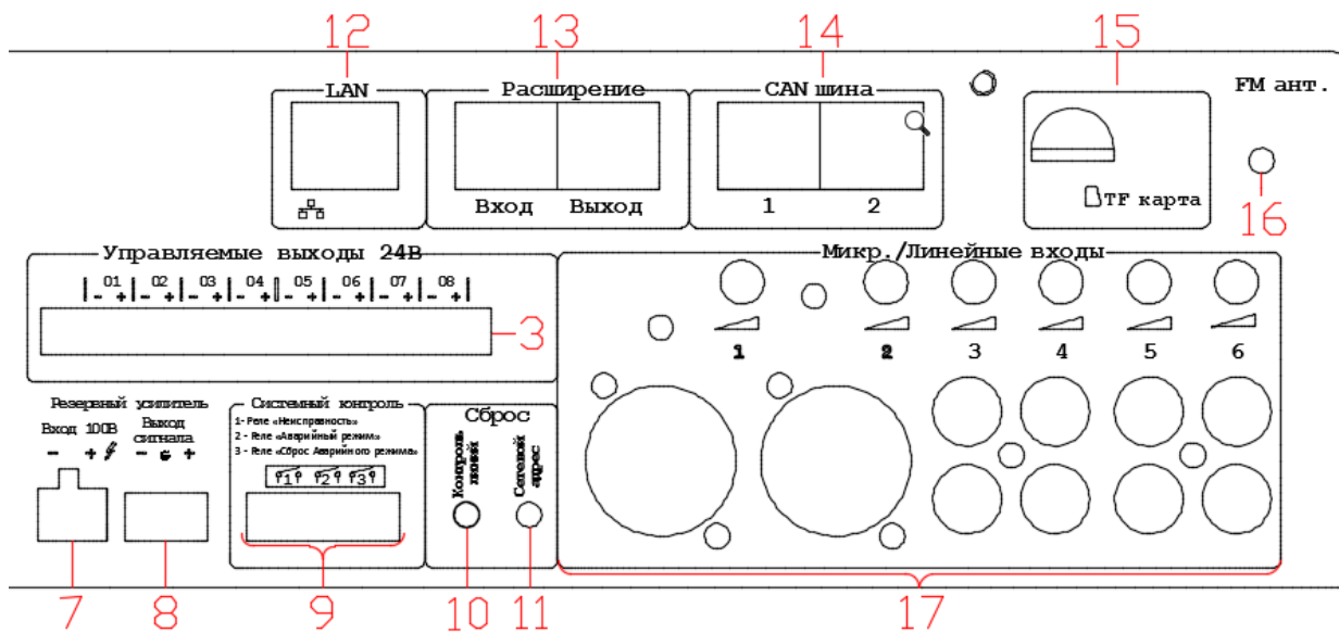
Рис. 2.1.3. Контроллер системы LPA-DUO-M (задняя панель)
