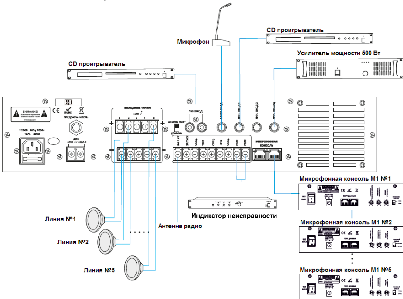
Рис. 2.1 Схема подключения
