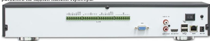
Рис. 1. Расположение разъемов на задней панели Прибора
