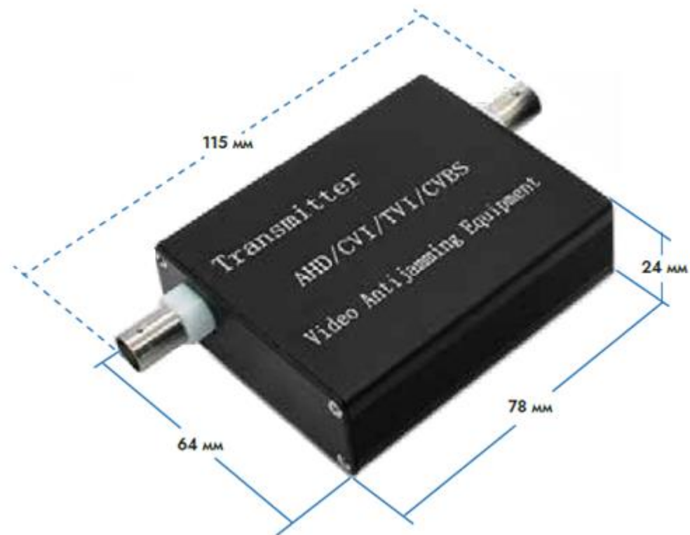
Рисунок 1. Габаритно-присоединительные размеры
