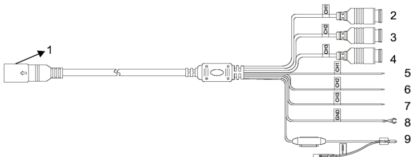
Рис. 4. Соединительный кабель.
