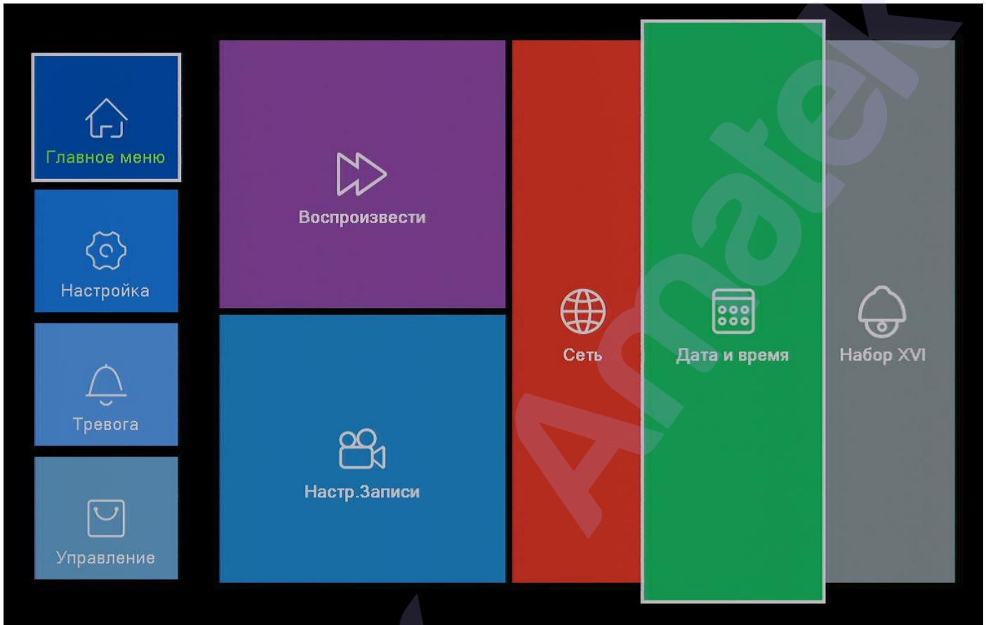
Рис. 4.1 Главное меню
