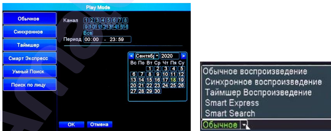
Рис. 3.6 Режимы воспроизведения
