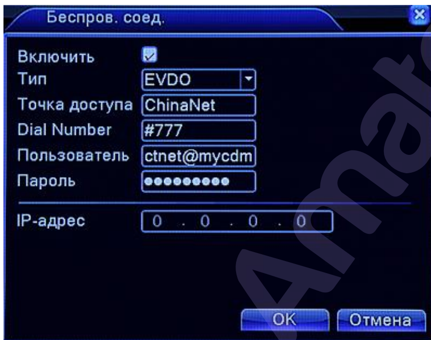
Рис. 4.12 Беспроводное соединение
