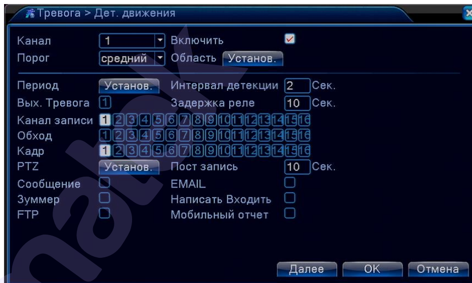
Рис 4.43 Обнаружение движения
