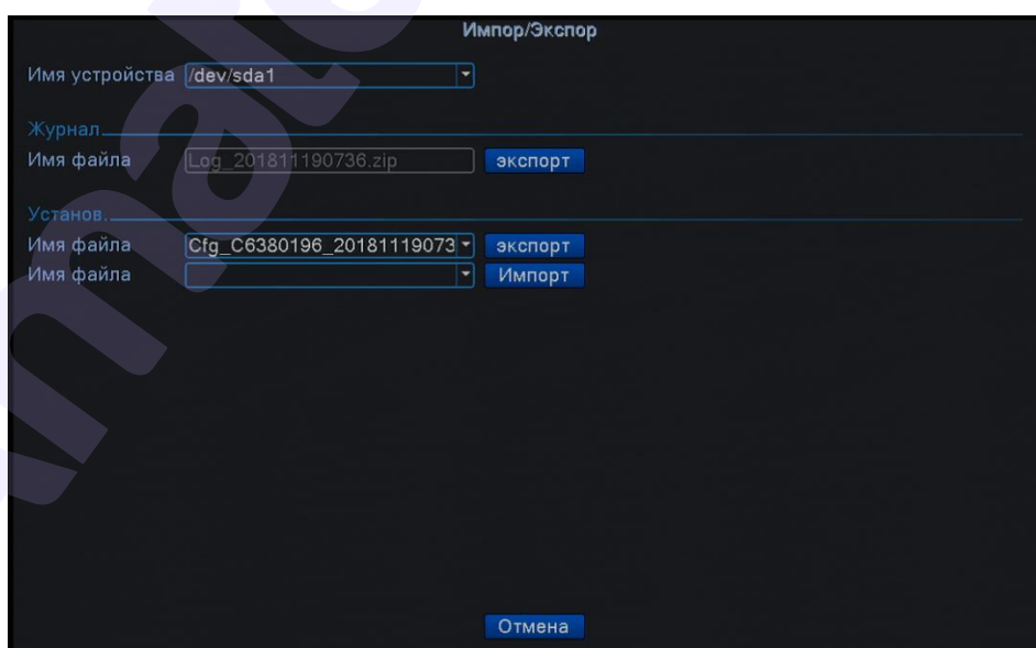
Рис 4.65 Импорт/экспорт
