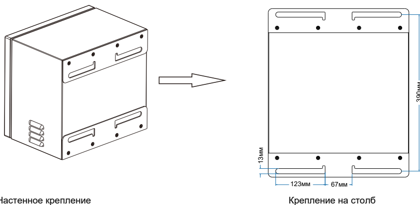
Настенное крепление
