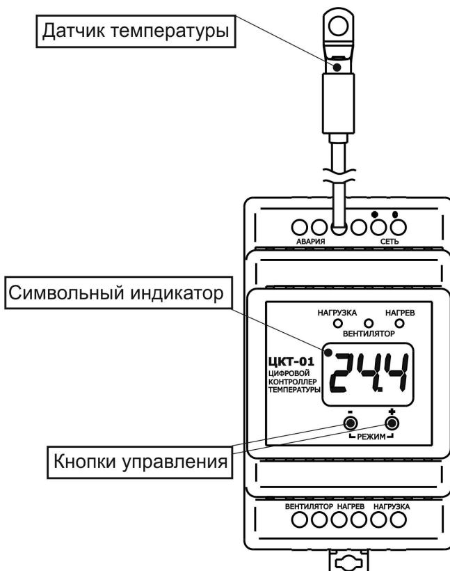
Рисунок 3 – общий вид ЦКТ
